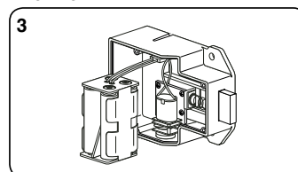
3 Das Batteriepaket aus dem hinteren Gehäuse nehmen.
